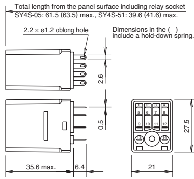
RY4S/RY42S
