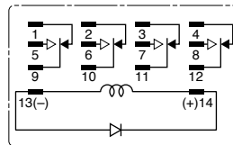
4PDT (RY4)
