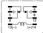
DPDT Slim (RY2/RM22)
