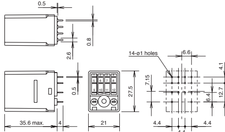
RY4V/RY42V
