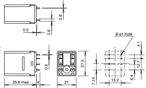
RM2V
